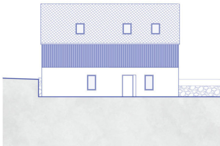
POHLED VÝCHODNÍ
