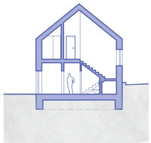
ŘEZ PŘÍČNÝ
