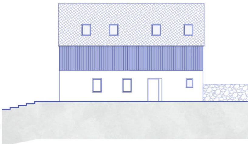
POHLED SEVERNÍ
