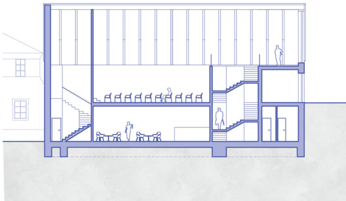
ŘEZ PODÉLNÝ
