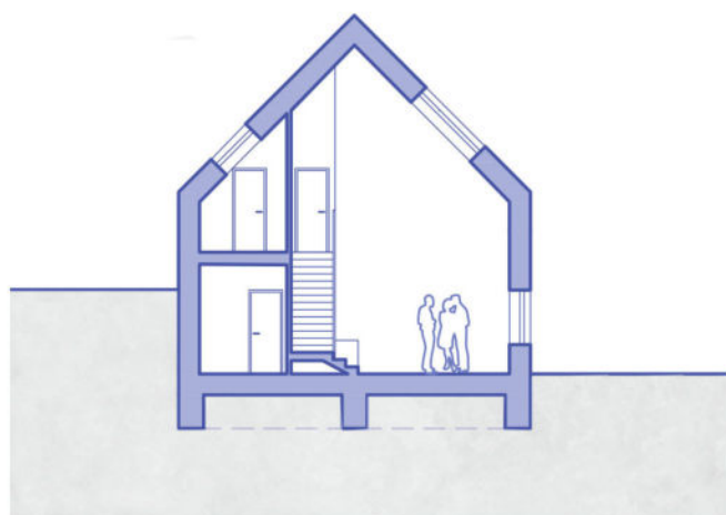
ŘEZ PŘÍČNÝ
