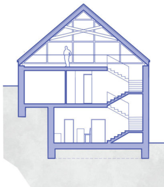
ŘEZ PŘÍČNÝ
