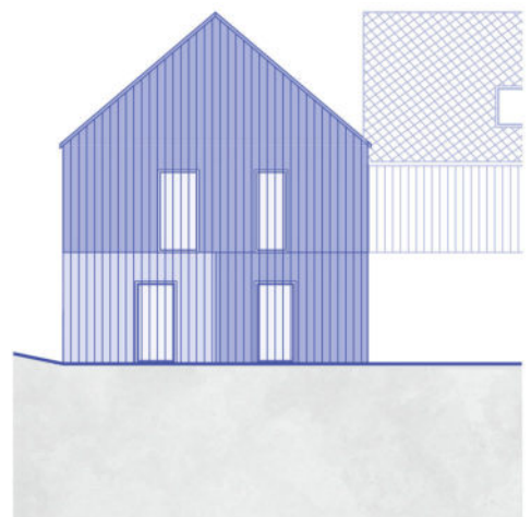
POHLED VÝCHODNÍ
